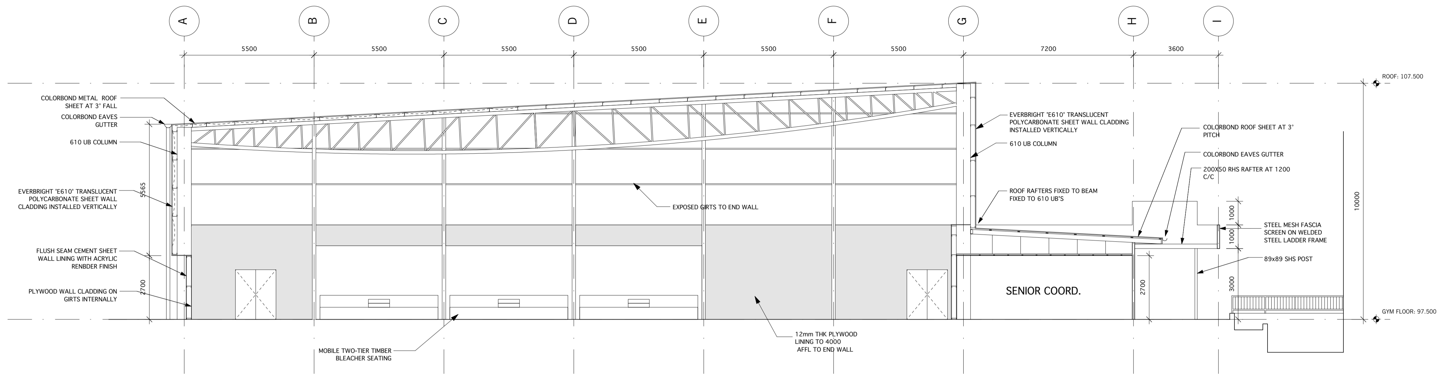
1 SECTION AA Scale: 1:100
